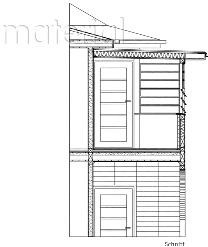
Schnitt
