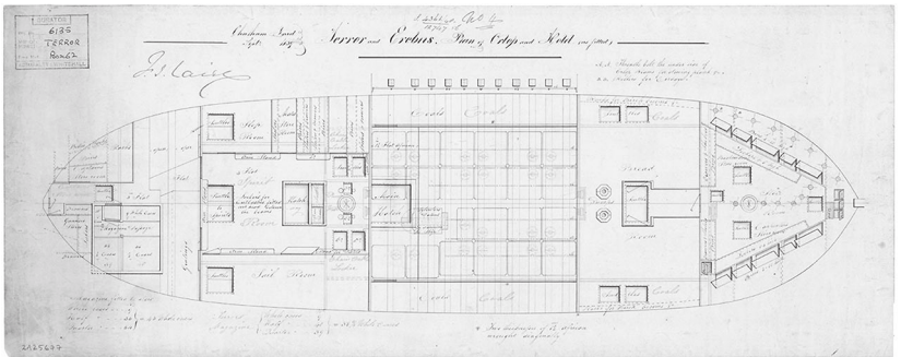
Zwei zeitgenössische Pläne zeigen die Seitenansicht einer typischen Bombarde (oben) sowie das Orlopedeck und die Lagerräume der Erebus und ihres Schwesterschiffes Terror (unten).
