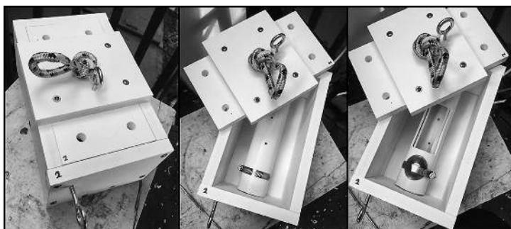
Testapparatur aus dem Versuch von Reid und Tousignant
