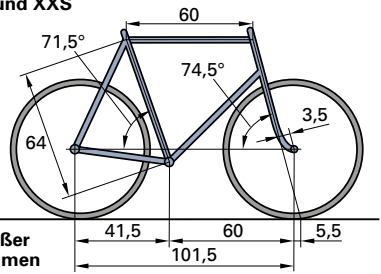
Rahmengenometrie für Renn- und Sporträder in XXL und XXS
