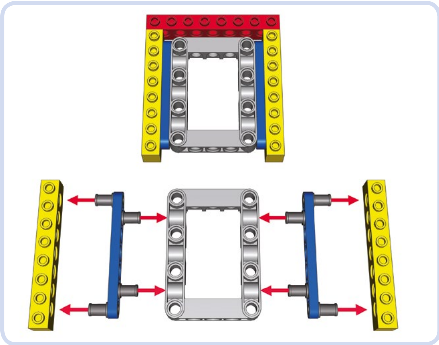
Abbildung 3-39: Dünne Balken (blau) und Dreiviertelstifte (dunkelgrau) können verwendet werden, um eine feste Verbindung zwischen Teilen geradzahligter und ungeradzahligter Länge zu bilden.
