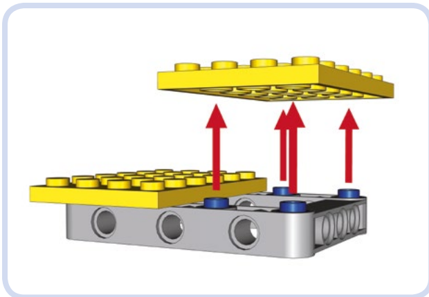
Abbildung 3-33: Werden halbe Stifte in Stiftlöcher eingeführt, funktionieren ihre überstehenden Enden wie Noppen. Steine und Platten können fest daraufgesteckt werden. Die genaue Ausrichtung können wir bestimmen, indem wir die Position der Halbstifte mit Bedacht auswählen.
