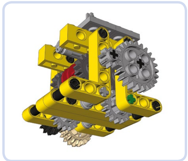
Abbildung 3-15: Dieses Getriebe habe ich aus noppenlosen Teilen zusammgebaut. Dazu musste ich planen, welche Stiftlöcher ich für Achsen verwenden wollte und welche für Stifte. Außerdem musste ich ermitteln, wie viele Verbindungen notwendig waren, um eine starre Struktur zu bekommen, und die durch ihre Form und Größe am besten geeigneten Teile sorgfältig auswählen.
