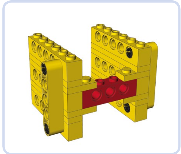
Abbildung 3-6: Der rote Stein wird zwar nicht direkt gesichert, aber durch die L-förmigen Eckplatten festgehalten. Diese Platten wiederum sind durch vertikale Steine gesichert.
