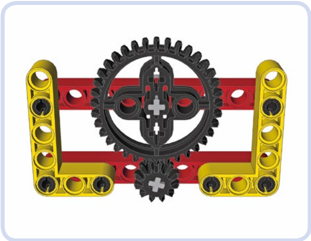
Abbildung 3-12: Teile, die über eine starre Verbindung zusammengehalten werden, benötigen gewöhnlich keine zusätzliche Sicherung, um auch bei Wirken eines Drehmoments zusammenzubleiben. Aufgrund der starren Verbindungen verhalten sich diese vier Bauteile wie ein einziges.
