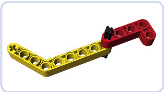
Abbildung 3-13: Wenn du zwei noppellose Elemente über Achslöcher verbindest, reicht eine einzige Achse aus, um eine starre Verbindung zwischen ihnen herzustellen. Diese Verbindung ist jedoch nicht so stark wie eine aus zwei oder mehr Stiften.
