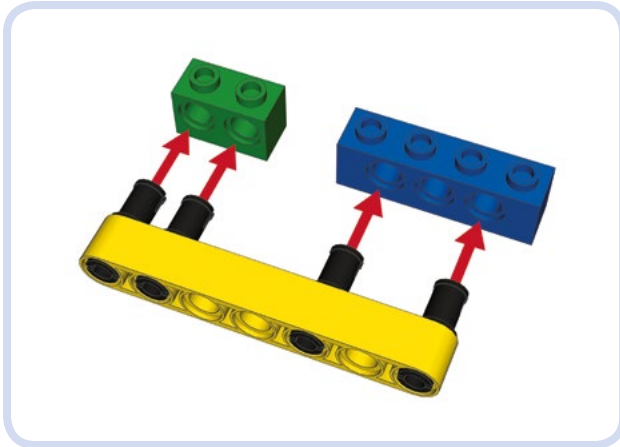
Abbildung 3-32: Balken können mithilfe von Stiften sehr leicht mit Steinen verbunden werden. Zur genauen Ausrichtung können wir sowohl reguläre Technic-Bausteine (blau) als auch Steine mit Stiftlöchern direkt unterhalb der Noppen verwenden.
