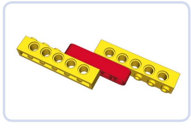
Abbildung 3-35: Diese Verbindung, bei der Noppen in die Stiftlöcher eines Balkens greifen, ist zwar stabil, wird aber als »falsch« betrachtet. Das liegt daran, dass die Stiftlöcher der beiden Steine nicht mehr um ein ganzzahliges Vielfaches einer Noppenlänge versetzt sind, wie es im vorherigen Beispiel der Fall war. Die Steine fluchten nicht.
