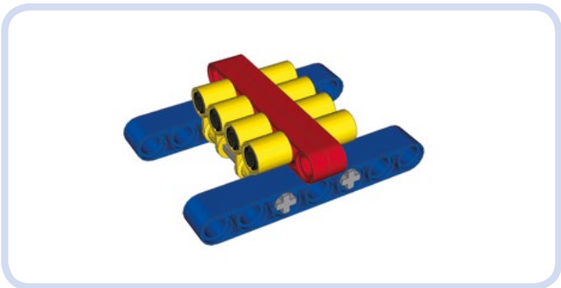
Abbildung 3-42: Verbinder (gelb) zur mittigen Ausrichtung eines sechs Noppen langen Teils (rot) an einer fünf Noppen langen Struktur (blau)
