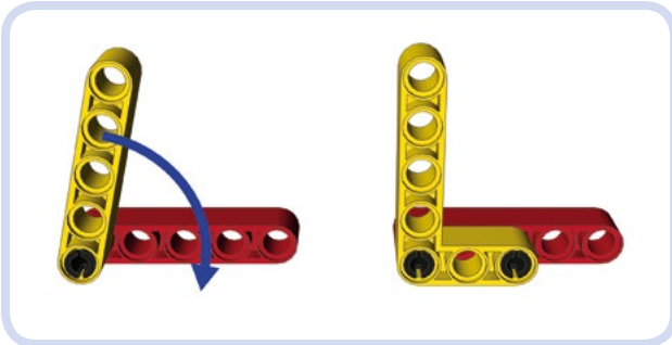
Abbildung 3-11: Eine nicht starre (links) und eine starre (rechts) Verbindung zwischen noppelosen Bauteilen im Vergleich. Bei der nicht starren Verbindung bleiben die Elemente zwar zusammen, aber ihre Orientierung zueinander kann sich ändern: Unabhängig vom Typ des Stifts für die Verbindung kann sich der gelbe Balken nach links oder rechts drehen. Bei einer starren Verbindung sind die Teile nicht nur verbunden, sondern auch fixiert, sodass sich ihre Orientierung zueinander nicht ändert.
