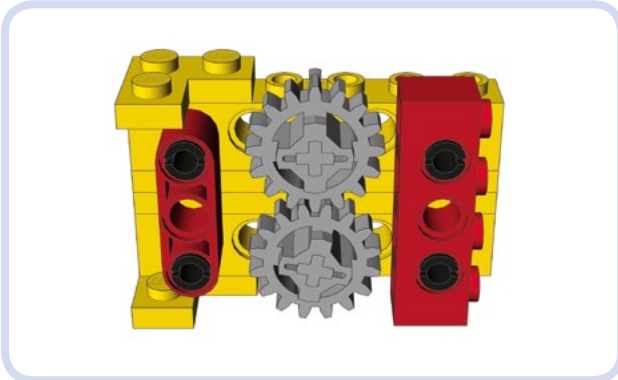
Abbildung 3-4: Zwei 1x6-Technic-Steine werden vertikal gesichert, um zu verhindern, dass sie sich lösen, wenn ein hohes Drehmoment auf die Zahnräder ausgeübt wird. Die noppenlose Klammer (links) braucht weniger Platz als die mit Noppen (rechts). Das lässt Raum für Platten oberhalb und unterhalb der beiden Steine oder für größere Zahnräder.
