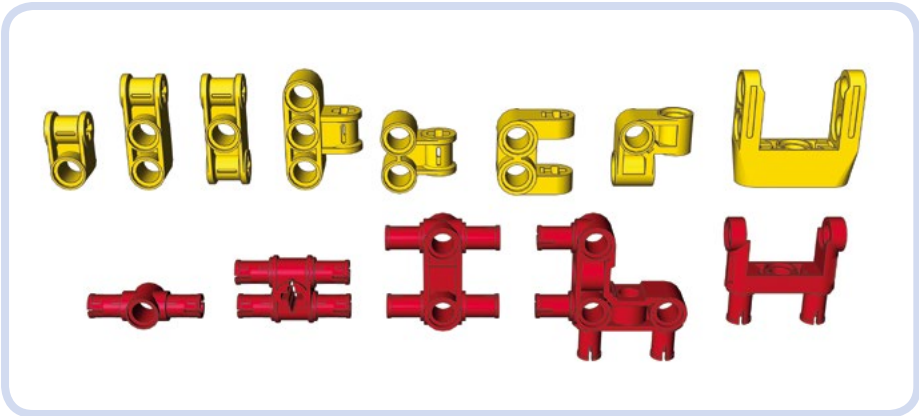
Abbildung 3-10: Die meisten noppelosen Verbinder weisen lediglich Stift- und Achslöcher auf (gelb), doch einige verfügen auch über integrierte Stifte (rot).
